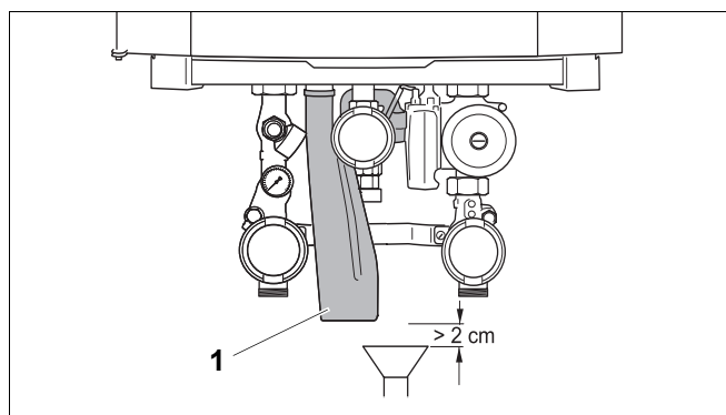
Рис. 11 Монтаж сифона
