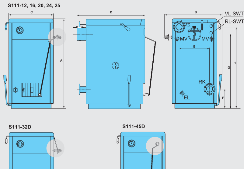
Рис. 3 Размеры и подключения
