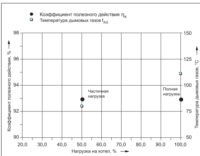
Диаграмма: Кoeffициент полезного действия и температура дымовых газов в зависимости от нагрузки на котел при средней температуре котловой воды 70 °C + температура дымовых газов, измеренная за прерывателем тяги
