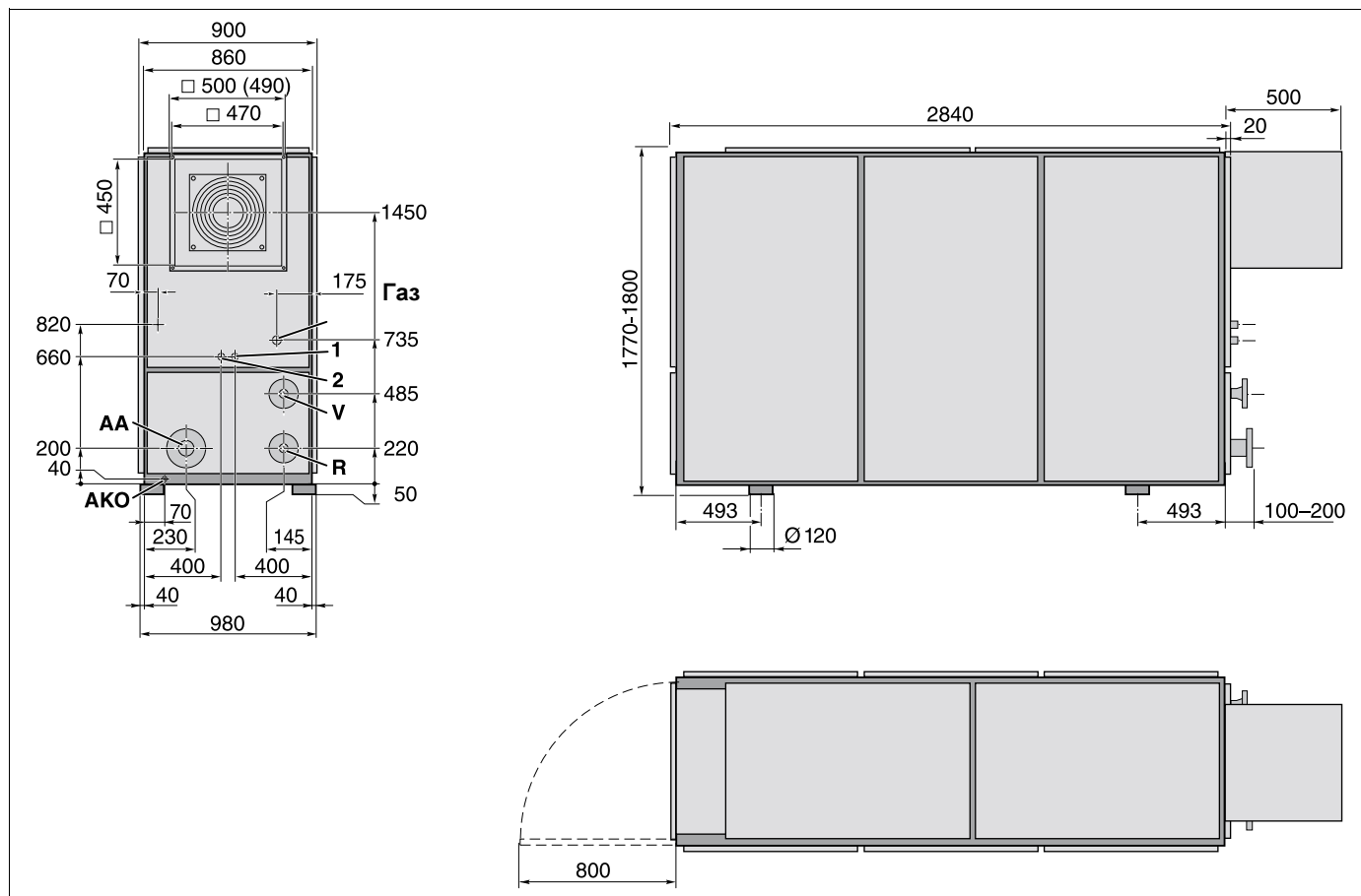
Рис. 4 Размеры (мм)
