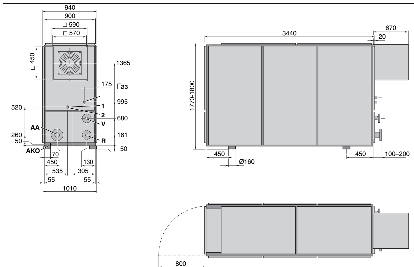
Рис. 4 Размеры (мм)
