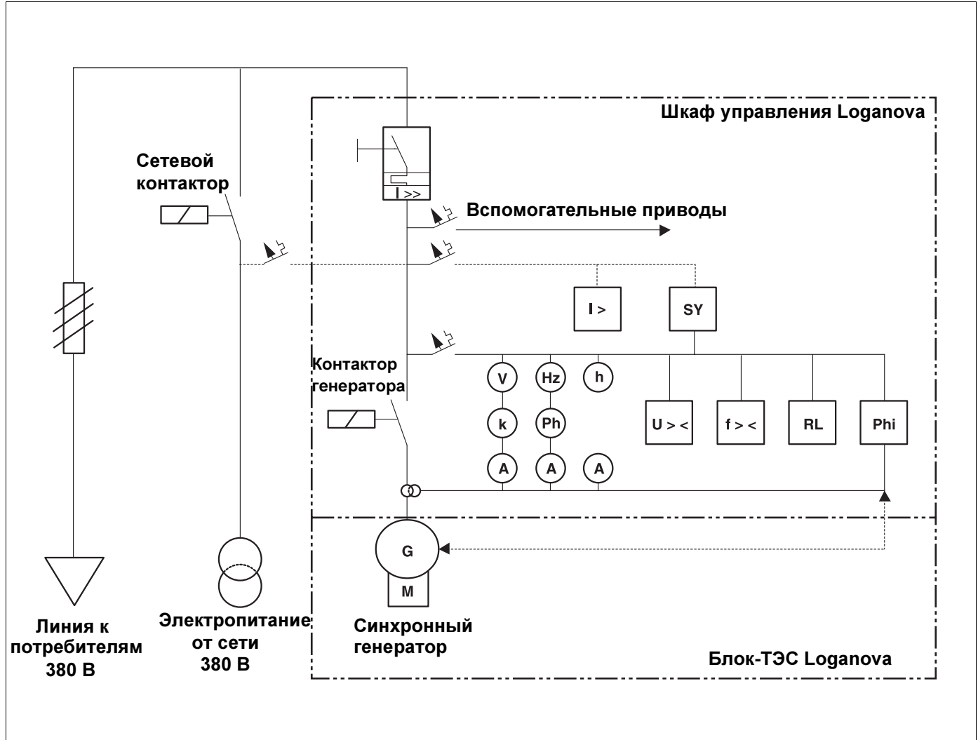
Рис. 3 Принципиальная схема электрических соединений для параллельной работы с сетью и для работы в качестве резервной сети
