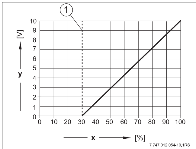
Рис.21 Клемма U_{BR}
